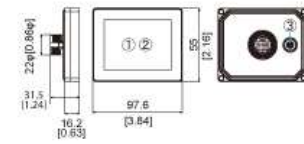
Display Module GP-4201TM
